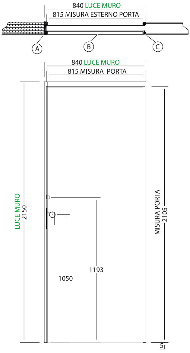
Porta Scorrevole (interno muro)
